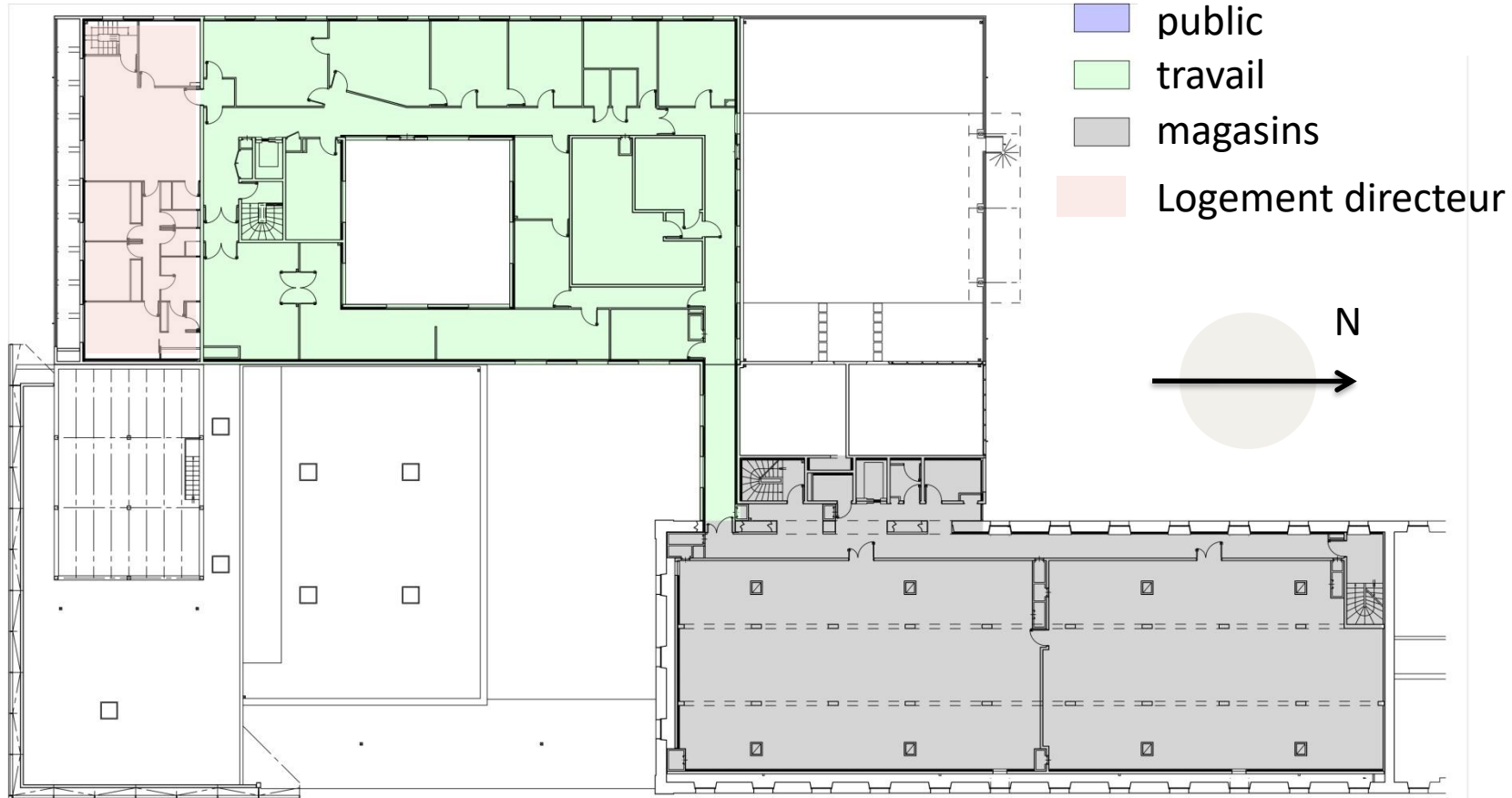
plan étage 1
